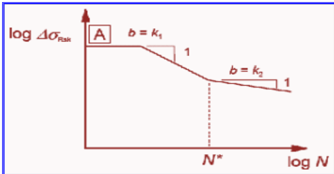
Figuur 9: basisvorm van de Wöhler kromme
