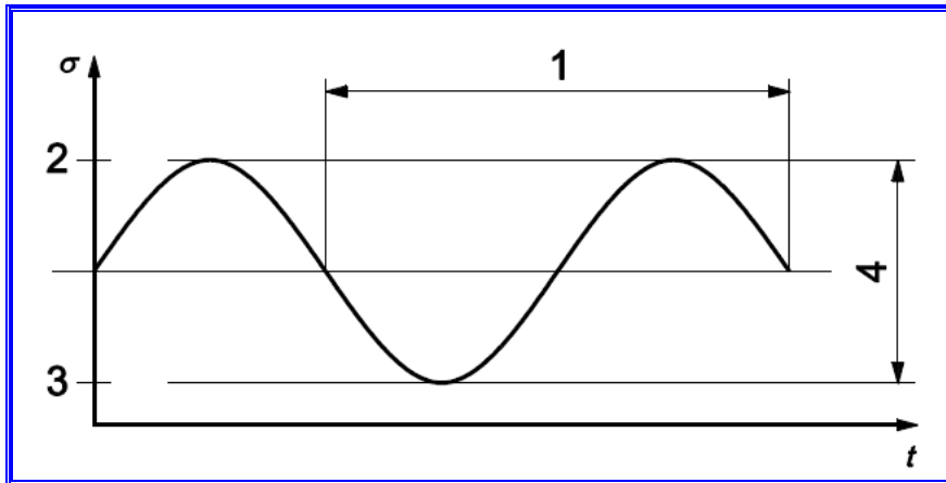
Figuur 7: Diagram van de lastcycli de vermoeiingsproef op groot aantal van cycli
