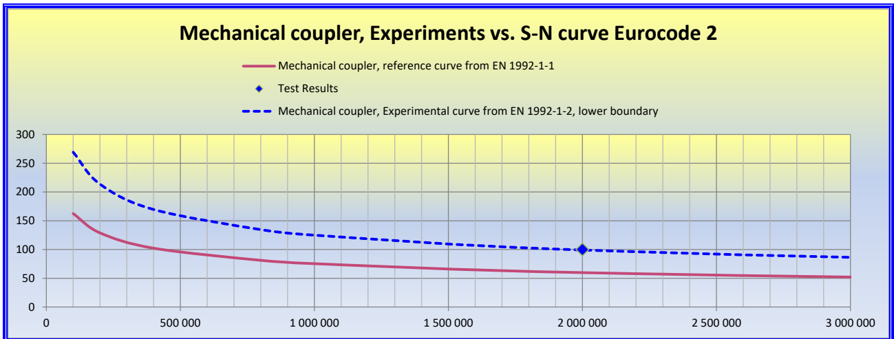
Figuur 3: Voorbeeld met een waarde van \Delta\sigma van 100 MPa voor twee miljoen cycli
