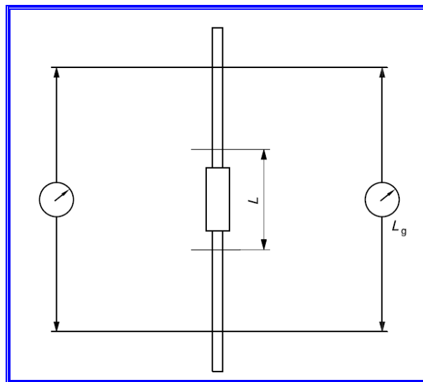
Figuur 4: Meetprincipe
