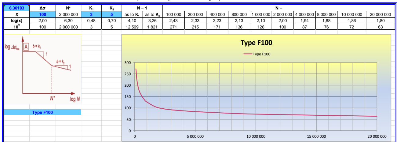
Figuur 10: Voorbeeld voor N^* = 2\,000\,000 , \Delta\sigma = 100 , k_1 = 3 , k_2 = 5
